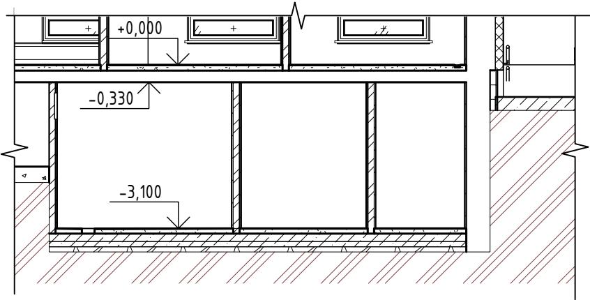
Разрез 1-1
